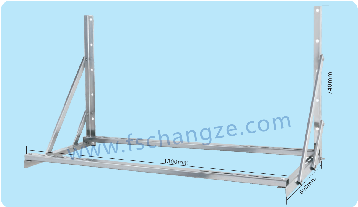
B311 5匹不锈钢组合吊架
