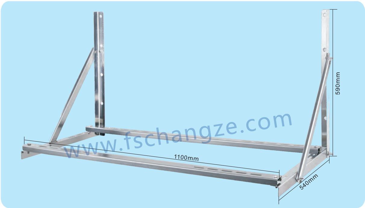
B309 3匹不锈钢组合吊架
